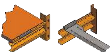
Reforço Z80 Z80 Reinforcement | Refuerzo Z80 | Renfort Z80
